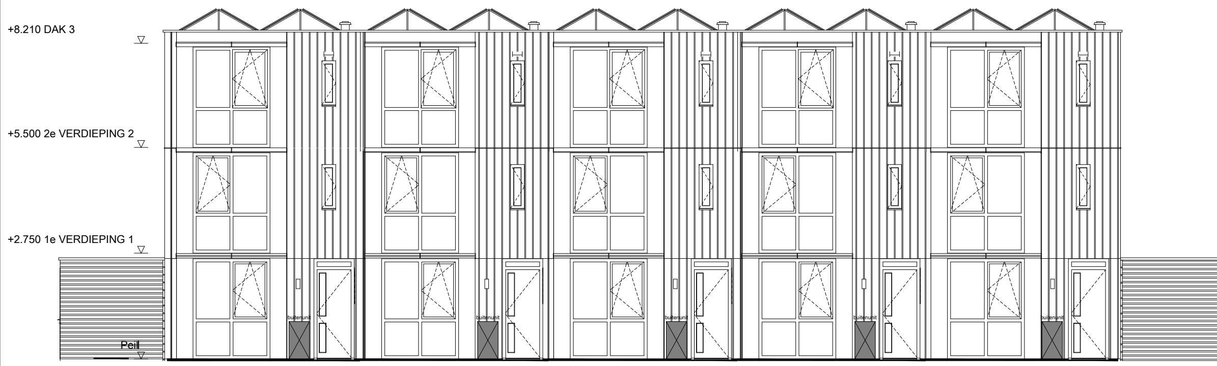
Voorgevel (oostgevel)
