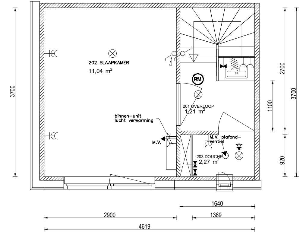
2e Verdieping
