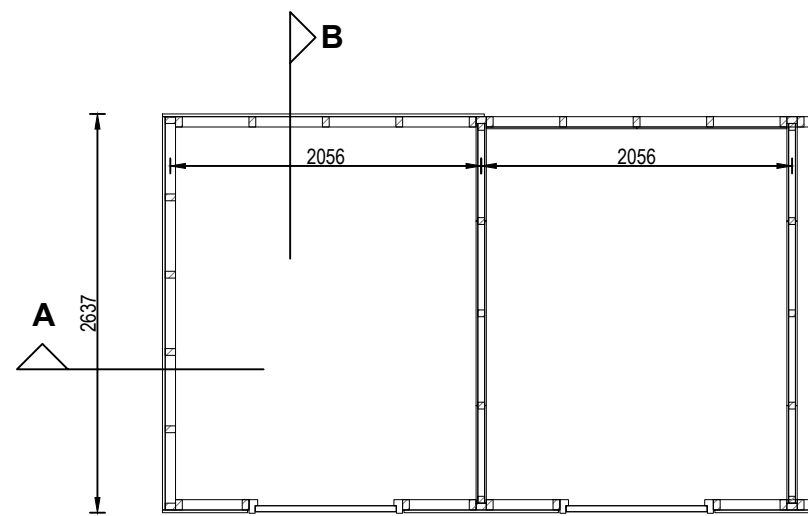
Plattegrond berging
