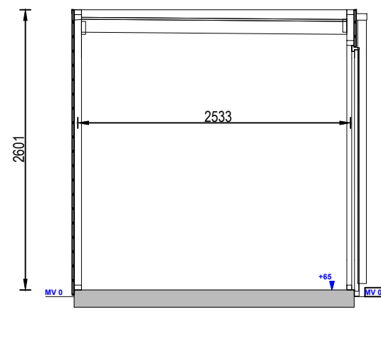
Doorsnede B
