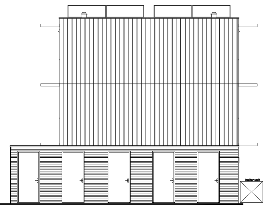
Zijgevel (zuidgevel)
