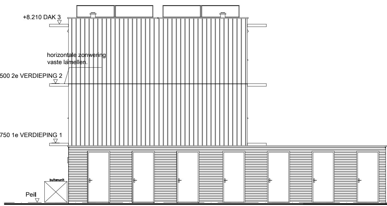
Zijgevel (noordgevel)
