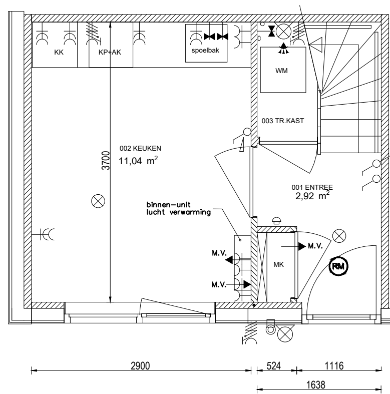
Begane grond
