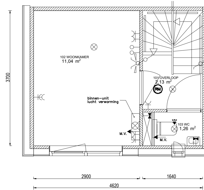
1e Verdieping
