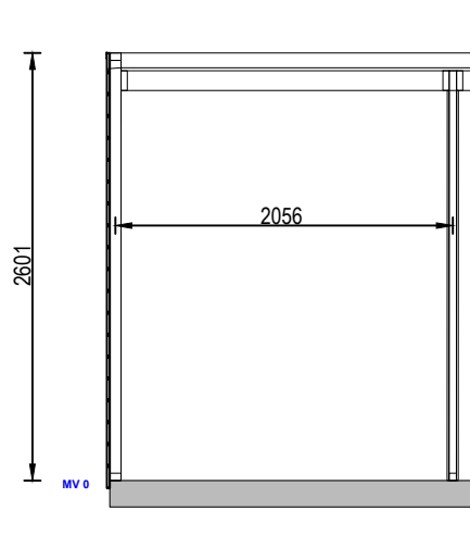
Doorsnede A
