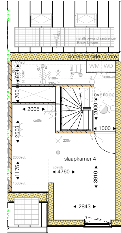
2e verdieping
