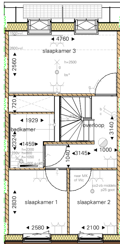
1e verdieping
