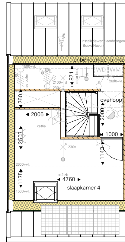
2e verdieping
