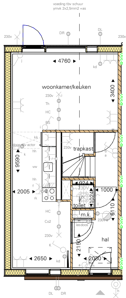
begane grond
