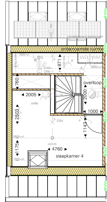
2e verdieping
