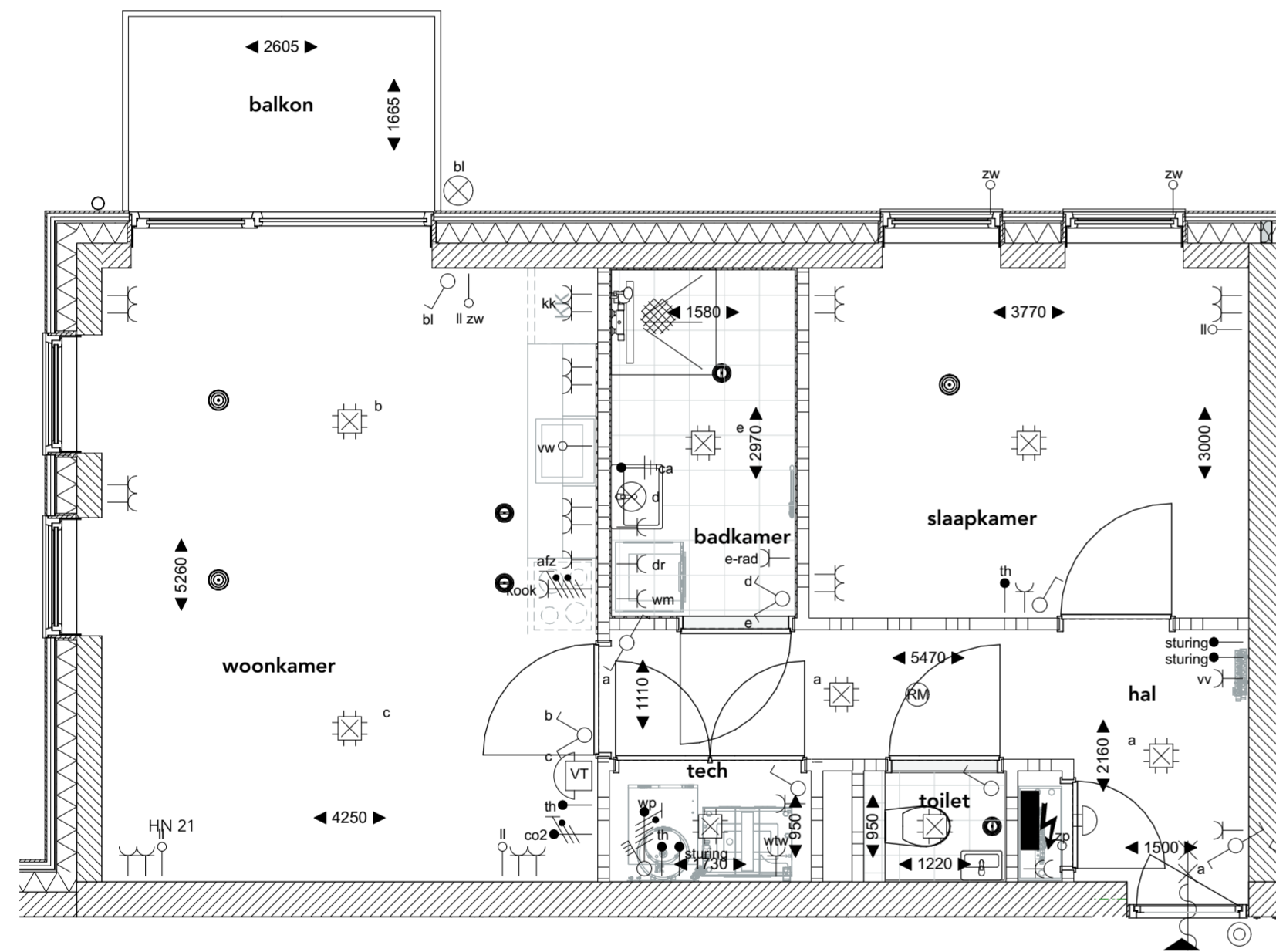
01 eerste verdieping 1:50
